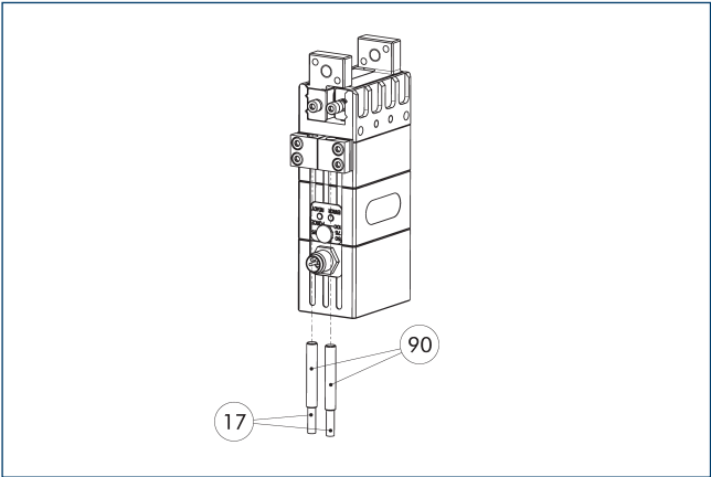
①⑦ ケーブルアウトレット ⑨⑩ 誘導型近接スイッチ
