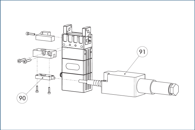
90 FPS-S センサー 91 FPS-F5 評価電子機器
