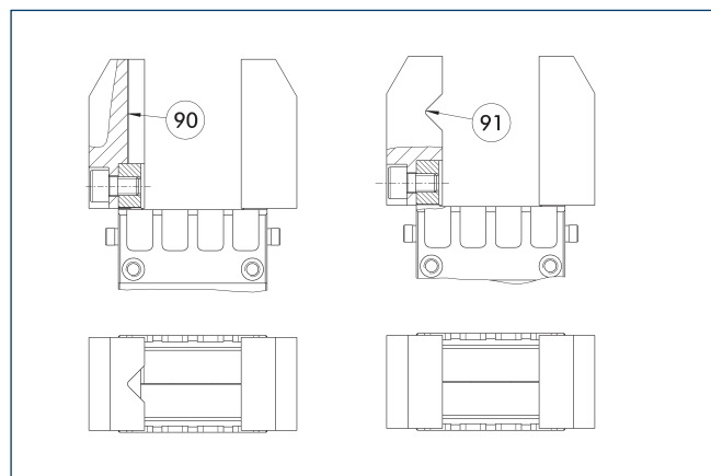
90 垂直に配置されたプリズム 91 水平に配置されたプリズム
