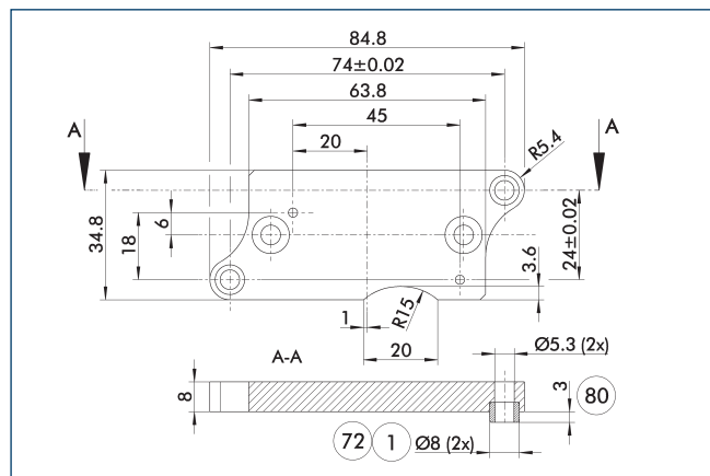
72 グリッパ接続 80 芯出しスリーブ穴の深さ (反対側)
