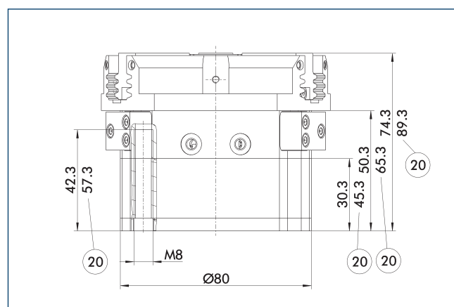
Цилиндр KVZ увеличивает усилие при открывании и закрывании. Второй подсоединенный последовательно поршень также увеличивает усилие в клиновом механизме. Обратите внимание на то, что захваты, оснащенные устройством поддержания захватного усилия, выше обычных.
