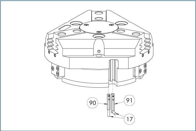
17 케이블 콘센트 90 센서 MMS 22-S-M8-PNP 91 센서 MMS 22-S-M8-PNP-SA
