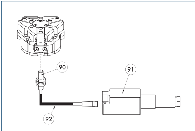
90 FPS-S 传感器
