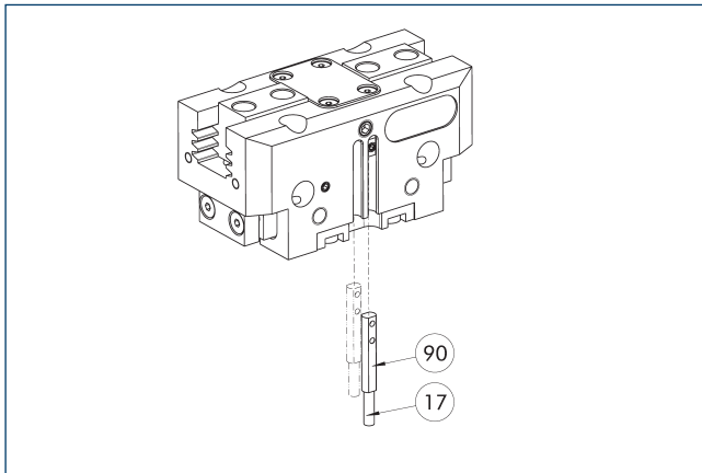
①⑦ Kabeluitgang
