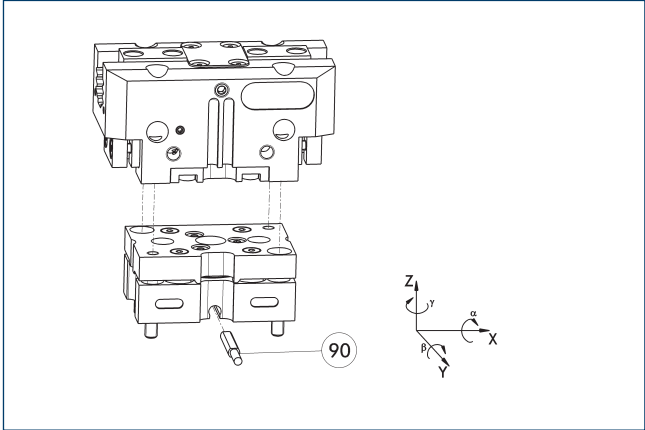
90 Bewaking van vergrendeling Grijpers kunnen direct worden gemonteerd zonder adapterplaat. Tolerantiecompensatie-eenheid en gripper hebben een identiek schroefverbindingsdiagram. Daarom kunnen de tolerantiecompensatie-eenheden later worden gemonteerd. Houd rekening met de bijkomende montagehoogte van de tolerantiecompensatie-eenheid. Voor details zie onze catalogus robotaccessoires.
