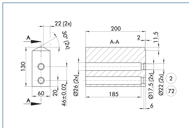
(72) Sede per boccia di centraggio
