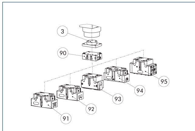
③ 어댑터 ⑨② 2조 평행 그리퍼 JGP-P ⑨③ SDV-P E-P 압력 유지 밸브 ⑨④ 2조 앵글 그리퍼 PWG-plus ⑨① 2조 평행 그리퍼 PGN-plus/ ⑨⑤ 2조 평행 그리퍼 PGB PGN-plus-P
