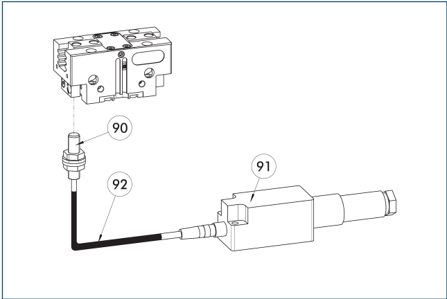
90 Sensor FPS-S 92 Prolongaciones de cable 91 Sistema electrónico de evaluación FPS-F5
