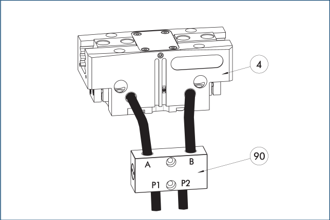
④ Pincés de préhension 90 Clapet anti-retour SDV-P
