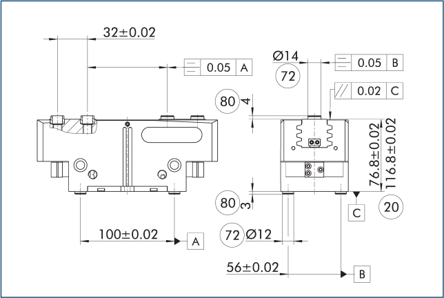
⑳ AS/ISバージョン向け ⑧ 芯出しスリーブ穴の深さ（反対側） ⑦ 芯出しスリーブ用
