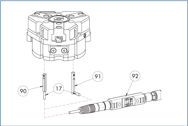
①⑦ ケーブルアウトレット ⑨① センサー MMS 22 ..-PI1-...-SA ⑨⑦ センサー MMS 22 PI1-... ⑨② コネクターティーチングツール ST
