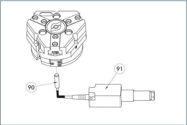
⑨① FPS-S センサー ⑨① FPS-F5 評価電子機器
