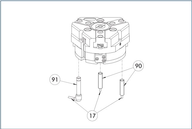
①⑦ ケーブルアウトレット ⑨① センサー IN...-SA
