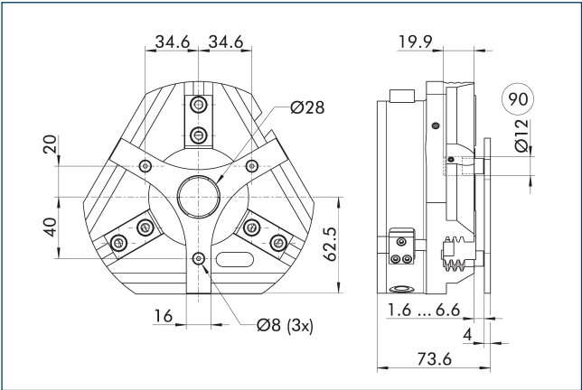
90 Geleidingspen
