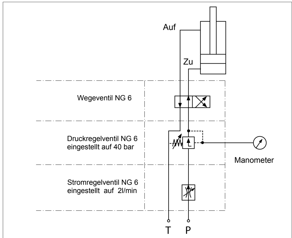
Schaltplan
