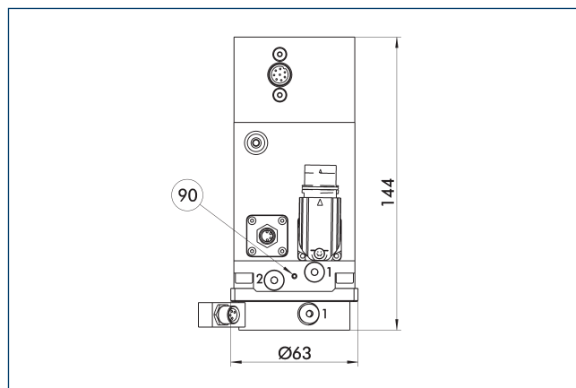
⑨⑩ Przyłącze powietrza do przedmuchu M3/6
