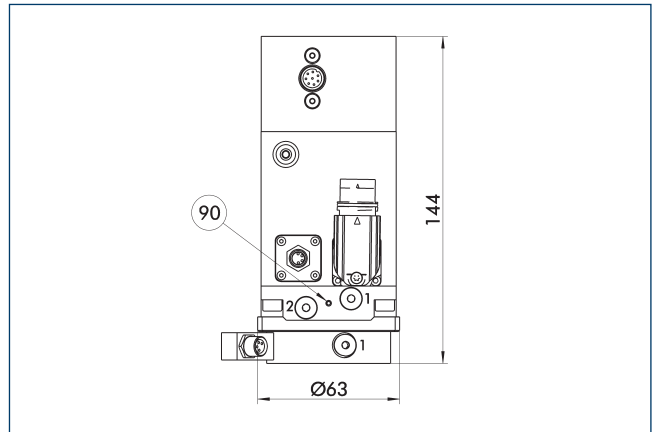
⑨⑩ M3/6 luchtspoelaansluiting
