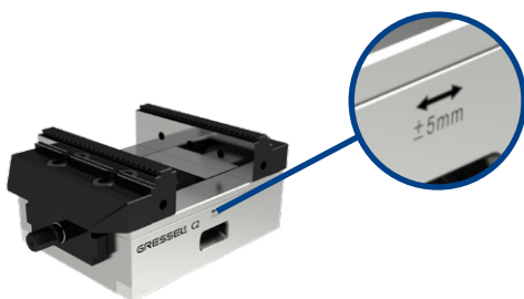
schwimmend – C2 125 L-160 floating – C2 125 L-160
