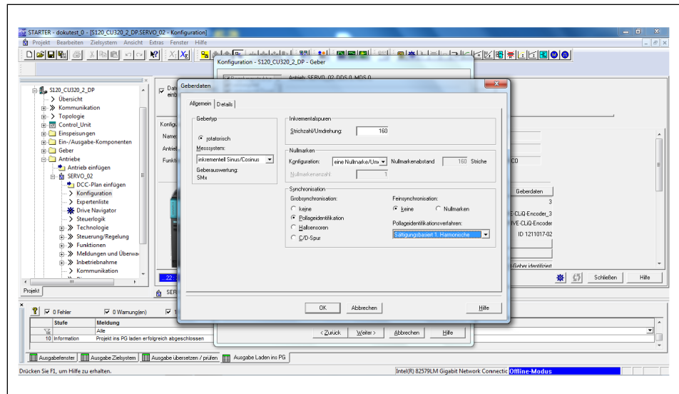
Encoder data for ERS135 (incremental)
