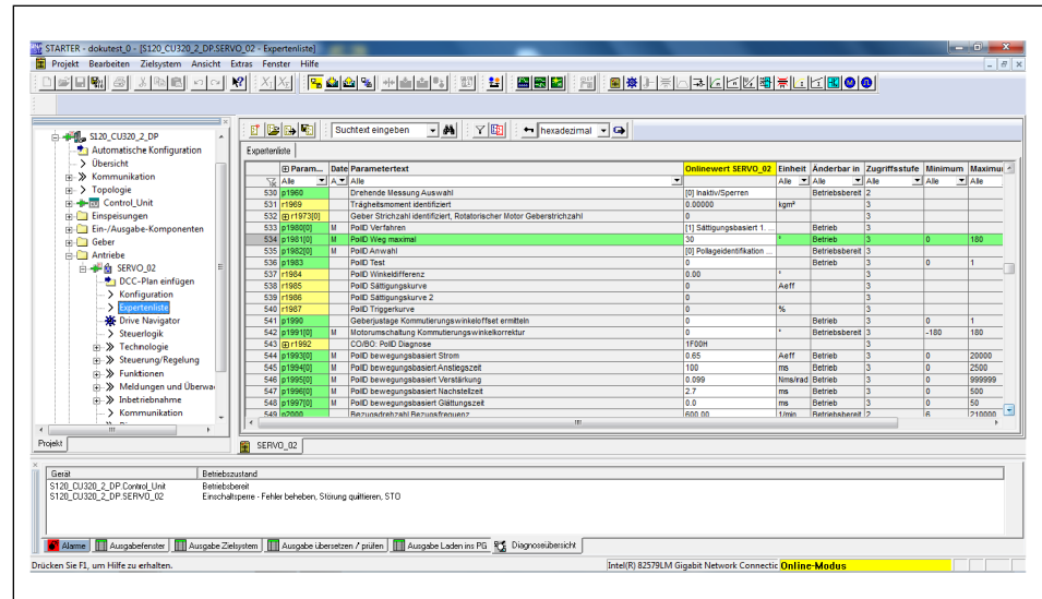
Expertenliste für das Parametrieren der Temperaturüberwachung bei Verwendung von absoluten Messsystemen
