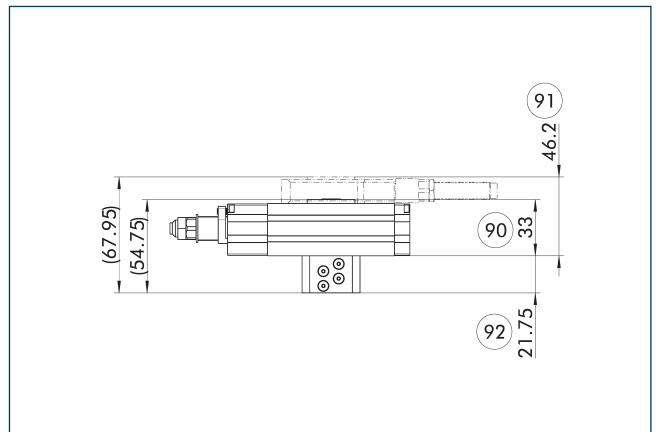
90 Gesamthöhe SRM Basis (Dämpfungsart H/E/S)
