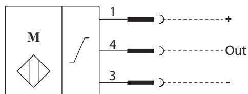
Anschlusschema
