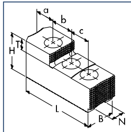
Aufsatzbacken hart, SP-HB Hard top jaws, SP-HB
