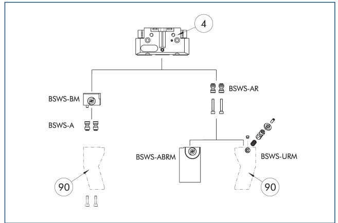
④ Greifer ⑨0 Kundenspezifische Greiferfinger
