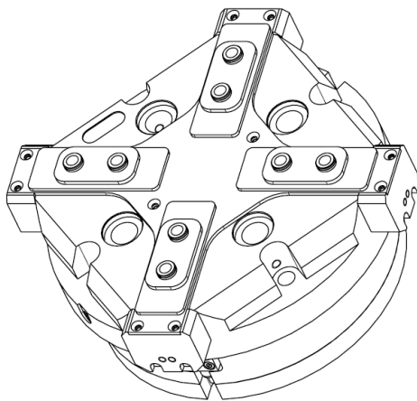
Abbildung 1: 4-Finger-Greifer mit Modifikation Staubabdeckung
