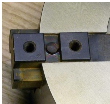
Abbildung 1: Greifer-Grundbacke ohne DLC-Beschichtung nach Verwendung in korrosiver Umgebung
