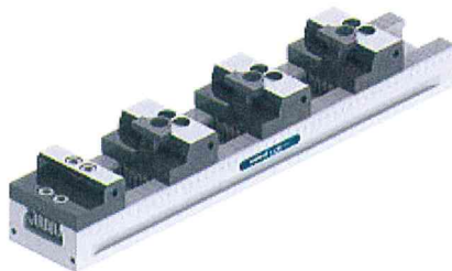
Mehrfachspannung auf engstem Raum: Mithilfe schlanker Backen lassen sich auf dem ›Kontec KSM2‹ mehrere Teile nebeneinander spannen.
