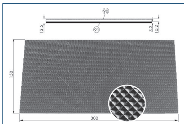
90 Almohadillas de elastómero 91 chuck base de acero inoxidable
