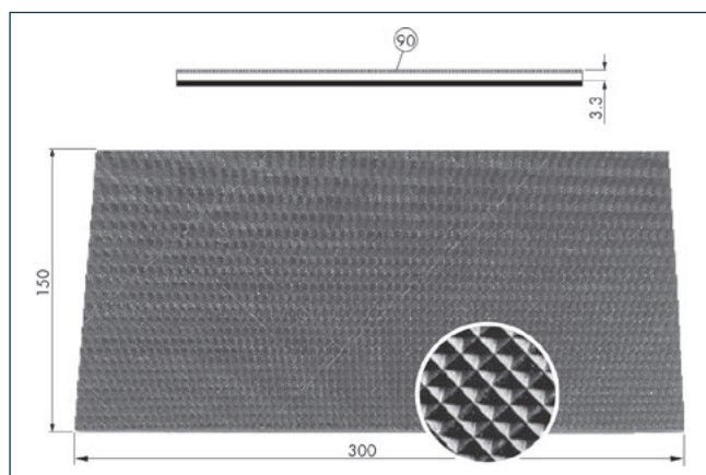
90 Almohadillas de elastómero
