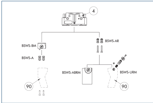
90 Kundenspezifische Greiferfinger
