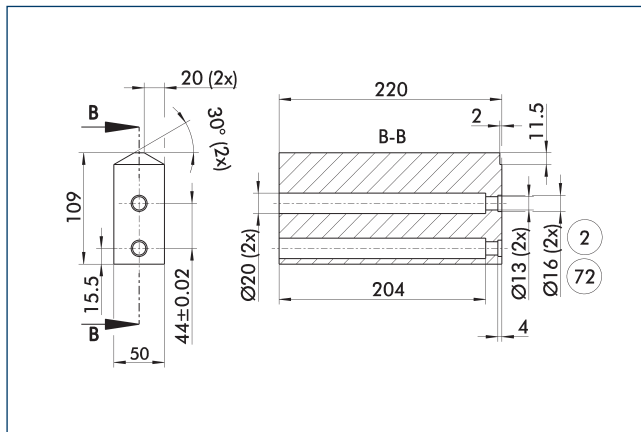
② Fingeranschluss
