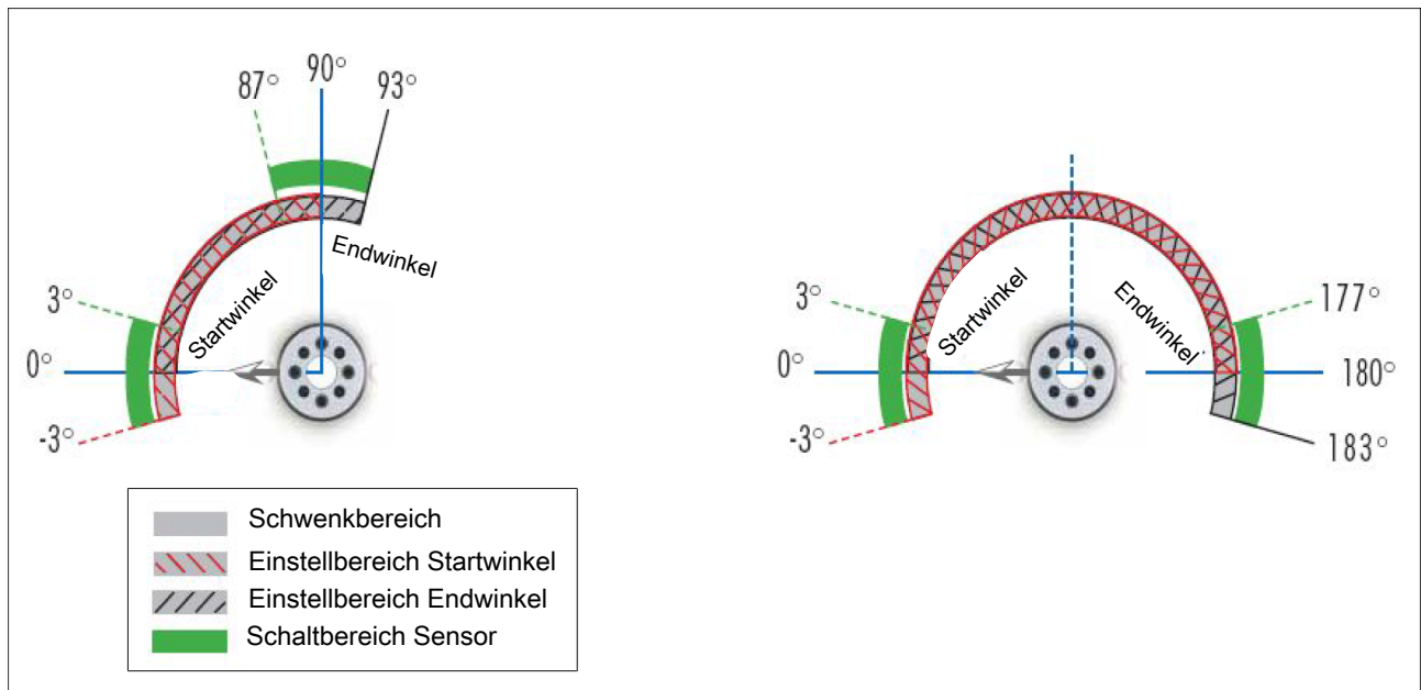
Schwenkwinkeleinstell- und Abfragebereich GSM
