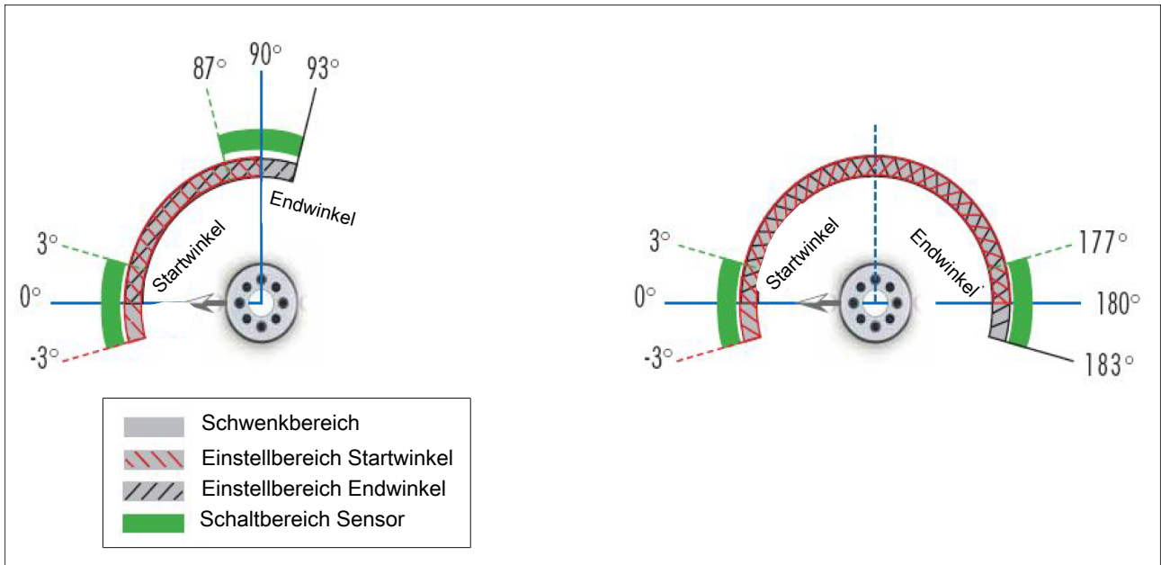
Schwenkwinklereinstell- und -abfragebereich mit GSM-Z
