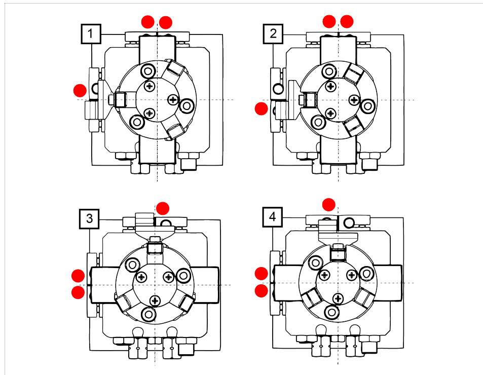
Prinzipdarstellung der induktiven Abfrage über INW 40 der GSM
