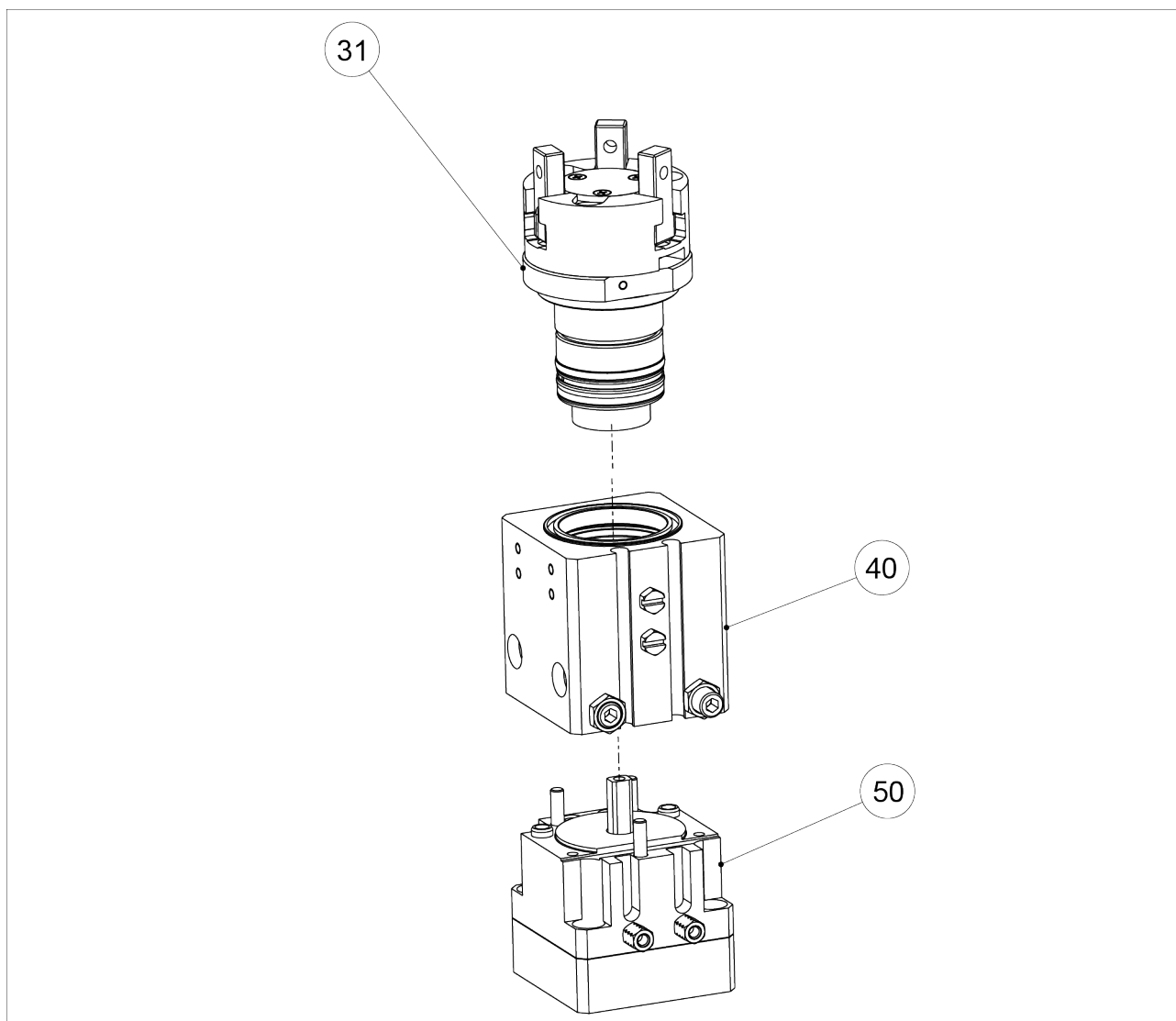
Zusammenbauzeichnung der Grundmodule
