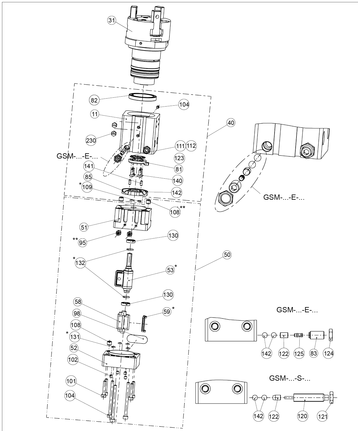
Zusammenbauzeichnung der Module DKM und FAN
