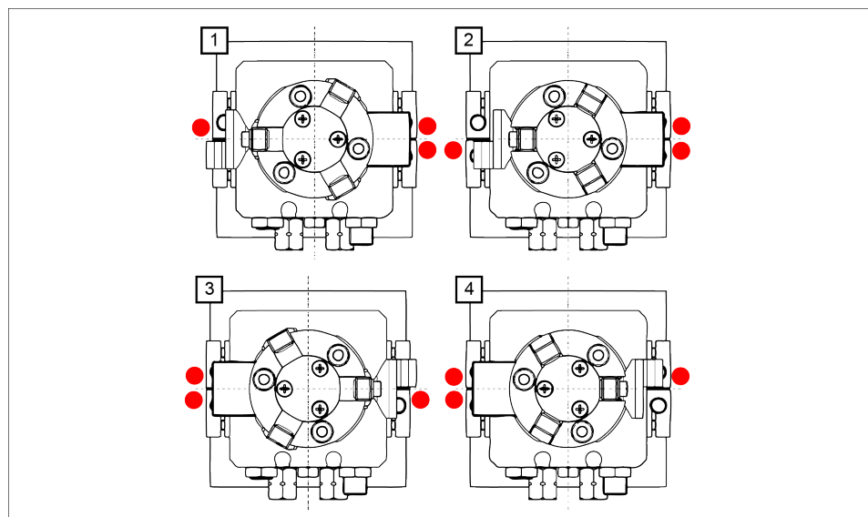
Prinzipdarstellung der induktiven Abfrage über INW 40 der GSM
