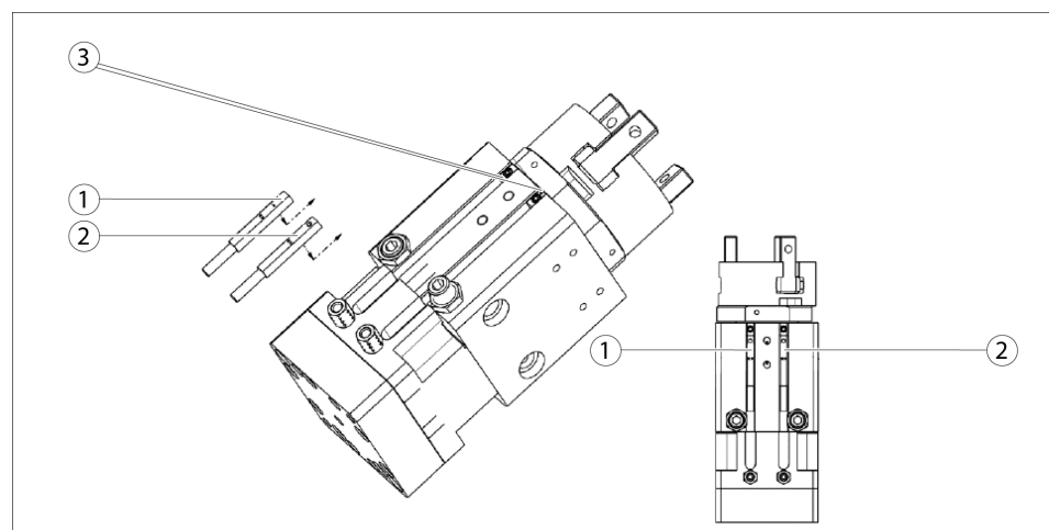
Position und Einbau der Magnetschalter MMS-P
