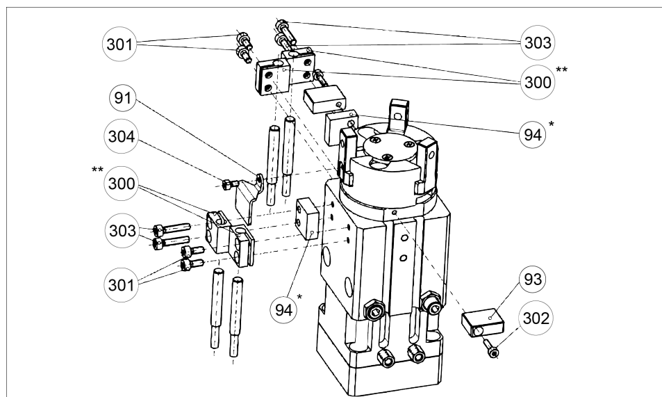
Zusammenbau der GSM 090-Varianten mit induktiver Abfrage
