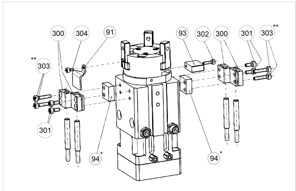
Zusammenbau der GSM 180-Varianten mit induktiver Abfrage
