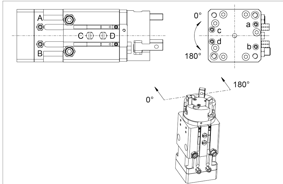
Pneumatische Anschlüsse
